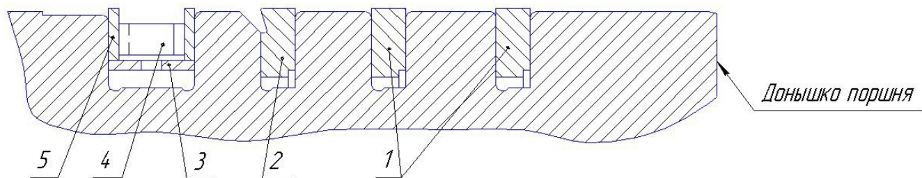
Схема установки поршневых колец
